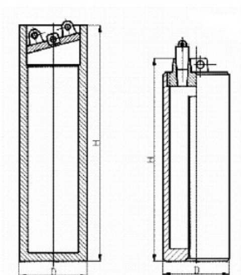
Общий вид пробоотборников ПО-1, ПО-2.
